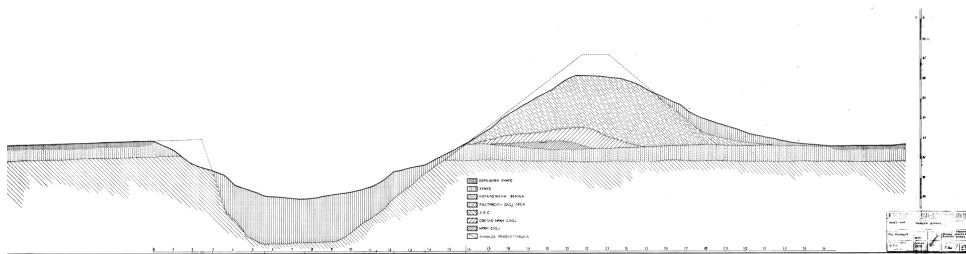
Ил. 5. Разрез на „Големия римски вал“ (по БУНАРЦИЌ 2005).
