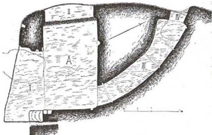
Обр. 17. Планъ на Долнитѣ Къшкове.
